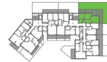
RZUT PARTERU
