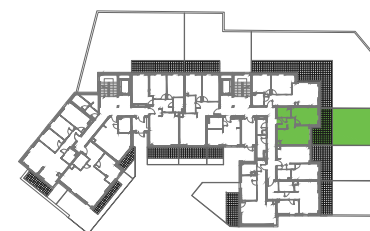
RZUT PARTERU
